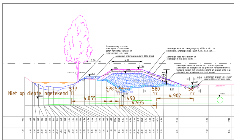
Figuur 1-2: Voorgenomen versterking ter plaatse van dijkvak 1, ter plaatse van AC-leiding.
