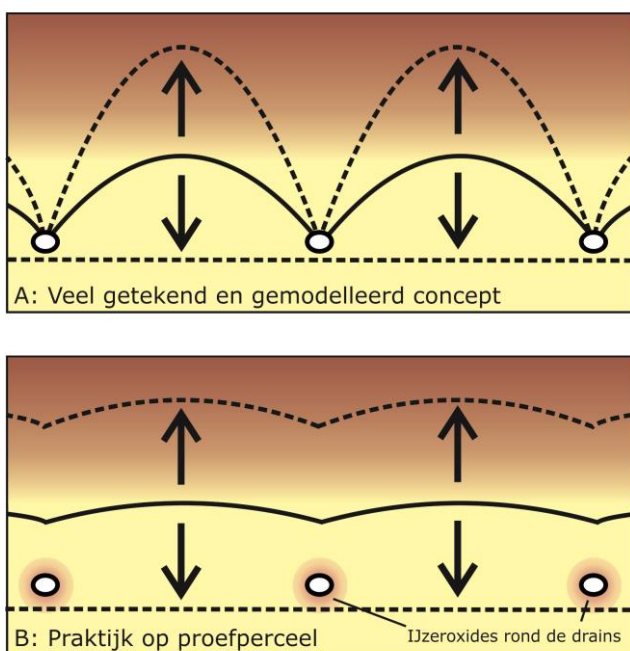
Figuur 5.1 Conceptuele weergave van het klassieke drainageconcept (A) en de praktijksituatie op het proefperceel met grondwaterstanden boven het drainniveau (uit Rozemeijer et al., 2012)
