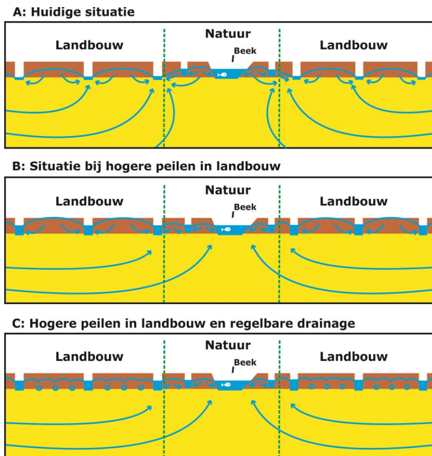
Figuur 1.2: Conceptuele voorstelling van de maatregel. A: Huidige situatie; lage grondwaterstanden in het landbouwgebied en daardoor geen kwel in natuur en lekkage naar het landbouwgebied. B: Herstel kwel en verminderen lekkage in natuur door peilopzet in landbouwgebied. C: Voorkomen van te hoge grondwaterstanden in landbouwgebied door peilopzet te combineren met drainage.
