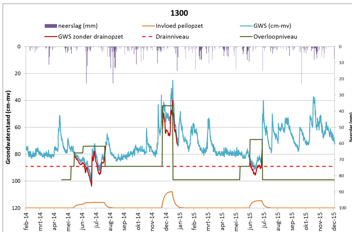
Figuur 4.2 Gemeten grondwaterstanden op locatie 1300 (meest westelijk, hoogst gelegen), berekende invloed van de peilopzet (referentie 120 cm = geen invloed) en berekende grondwaterstand zonder peilopzet.
