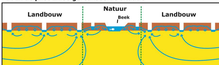
Figuur 5.2: Conceptuele voorstelling van de maatregel (zie ook hoofdstuk 1) met toegevoegd situatie D: De in de pilot Exloo gerealiseerde situatie. Door de geringe peilopzet verschilt die nauwelijks van de uitgangssituatie (A).
