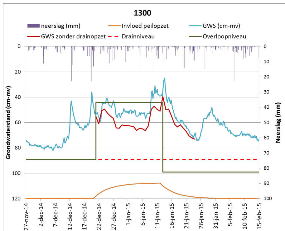
Figuur 4.3 Effect van extra peilopzet tijdens een proef in de winter van 2014/2015. Gemeten grondwaterstanden op locatie 1300, berekende invloed van de peilopzet (referentie 120 cm = geen invloed) en berekende grondwaterstand zonder peilopzet.
