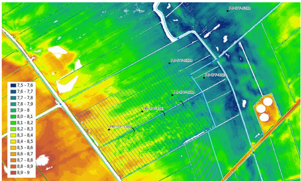
Figuur 3.2 Maaiveldhoogte, ligging drainage, peilbuizen en stuwen op het proefperceel.
