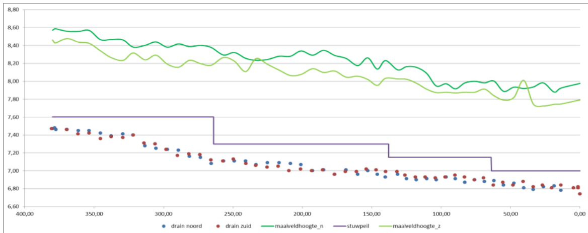
Figuur 3.5 Hoogteligging drainbuizen ten opzichte van maaiveld en de hoogte van een opgezet stuwpeil.
