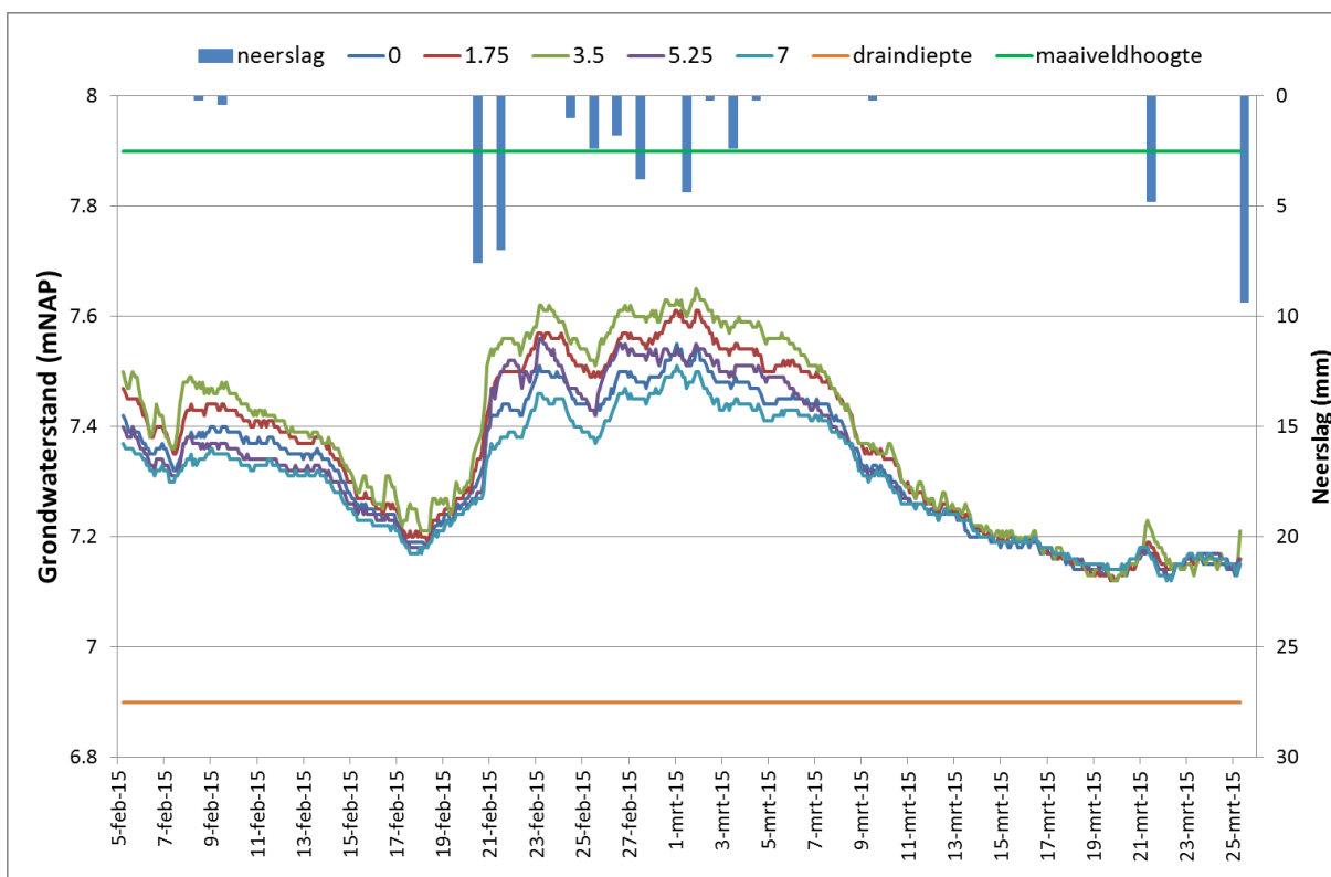
Figuur 4.4 Gemeten grondwaterstanden voor het bepalen van de opbolling tussen de drains; grondwaterstanden bij de drains (op 0 en 7m) en op 1.75, 3.5 en 5.25 m tussen de drains in.
