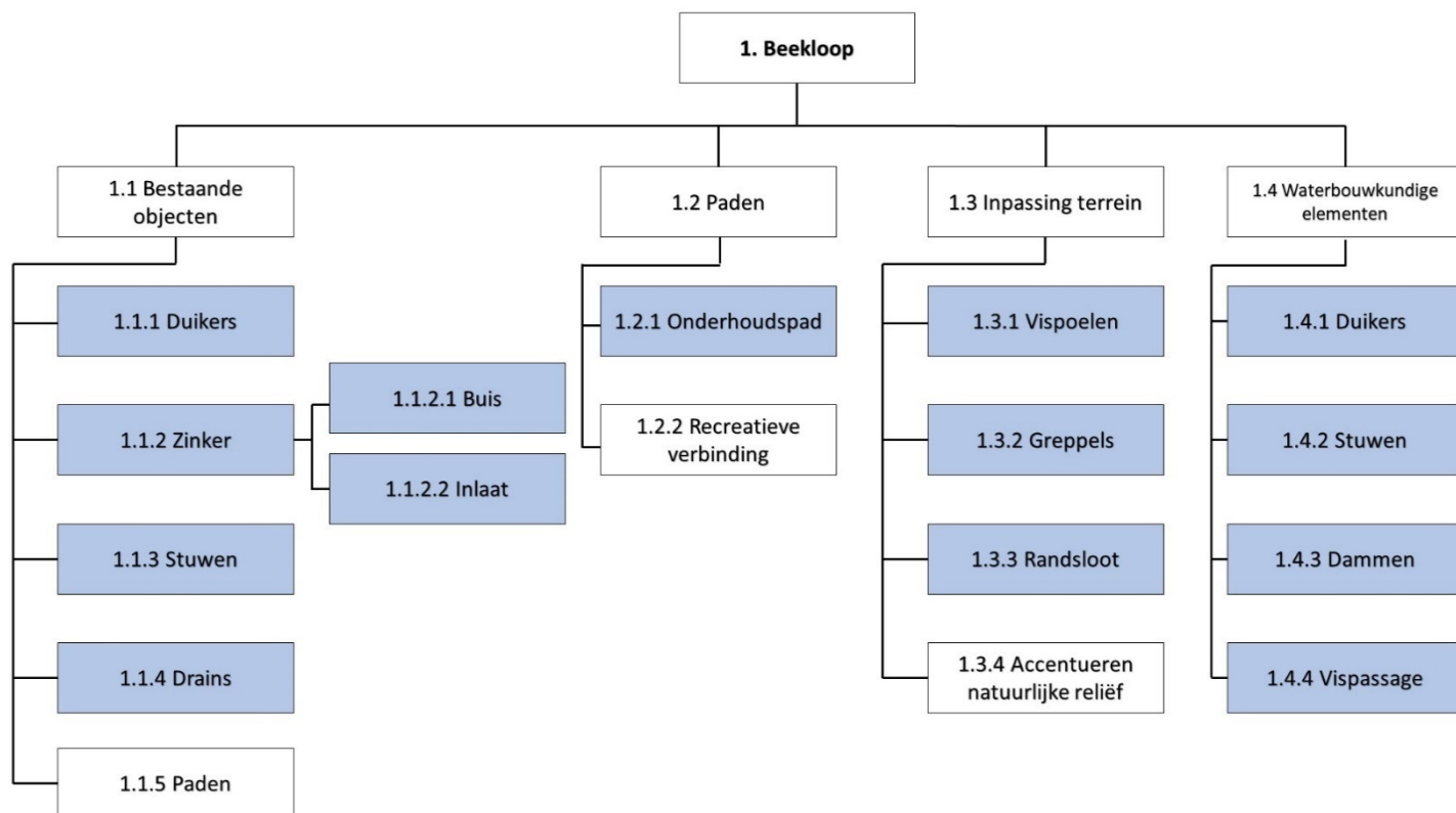
Figuur 6: Objectenboom
