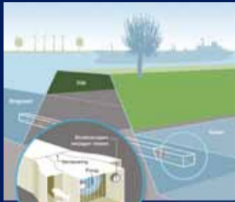
"Manshanden" gemaal vispassage bij gemaal Oude Aa.
